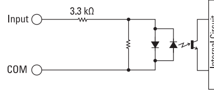
FC4A-N08B1, FC4A-N16B1
